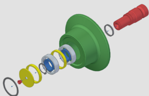
Zellenbandrolle mit Schmiernippel
